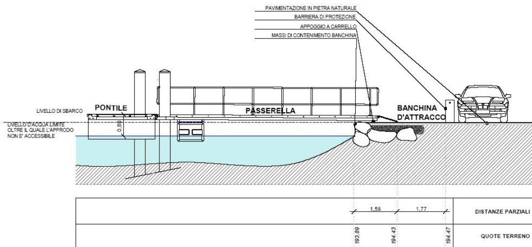
SEZIONE 1-1
